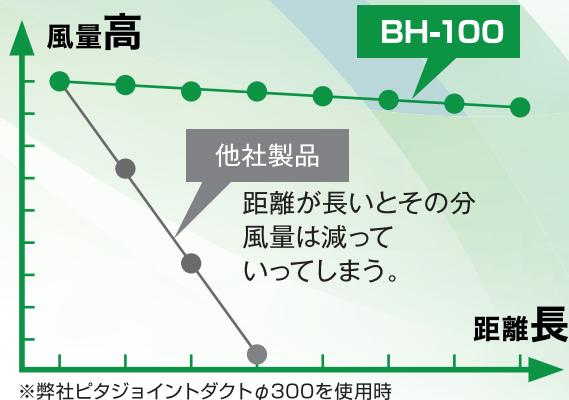
長距離ダクトに対応した高圧ブロワ
